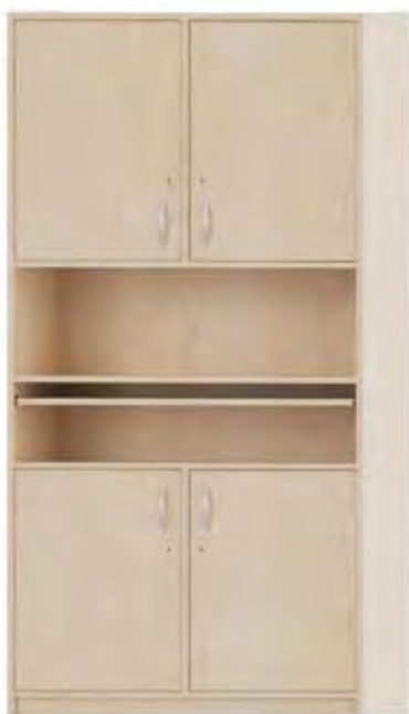
Hochschrank unten: Doppeltür abschließbar, Mittelwand, je 1 Einlegeboden mittig: offen mit ausziehbarer Schreibplatte oben: Doppeltür abschließbar, Mittelwand, je 1 Einlegeboden B/H/T 102 x 220 x 40 cm
